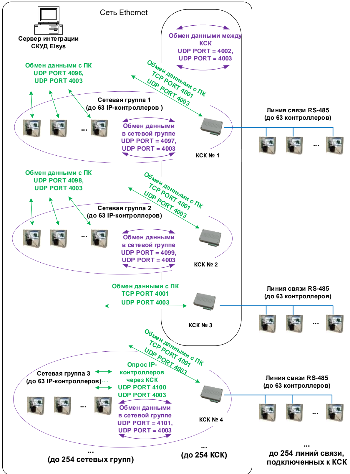
Рисунок 3. Использование КСК Elsys-NG-Net II в составе СКУД Elsys в обычном режиме (режим защищённого сетевого mTLS-соединения выключен)
